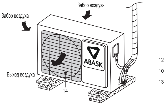
Внешний блок
