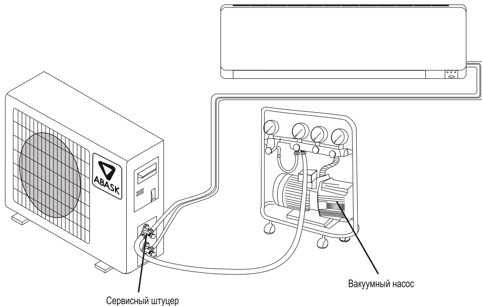
Сервисный штуцер
